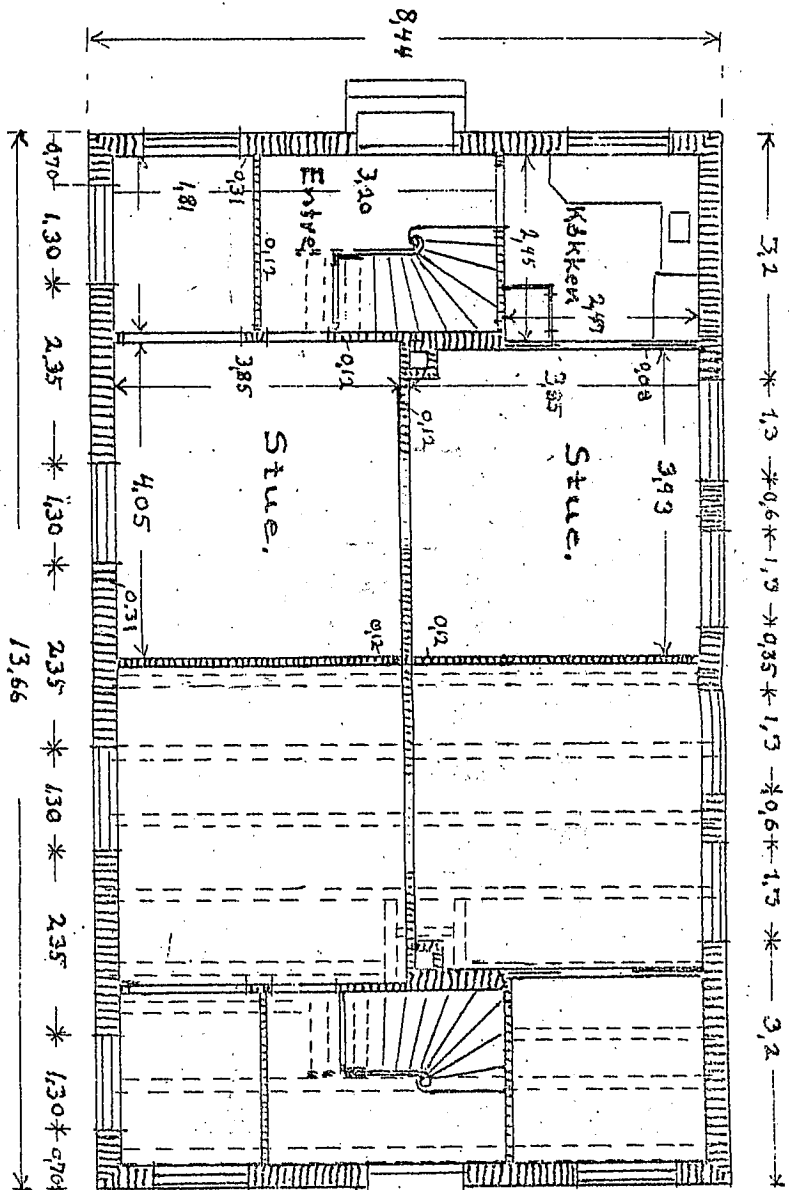
Stueplan
